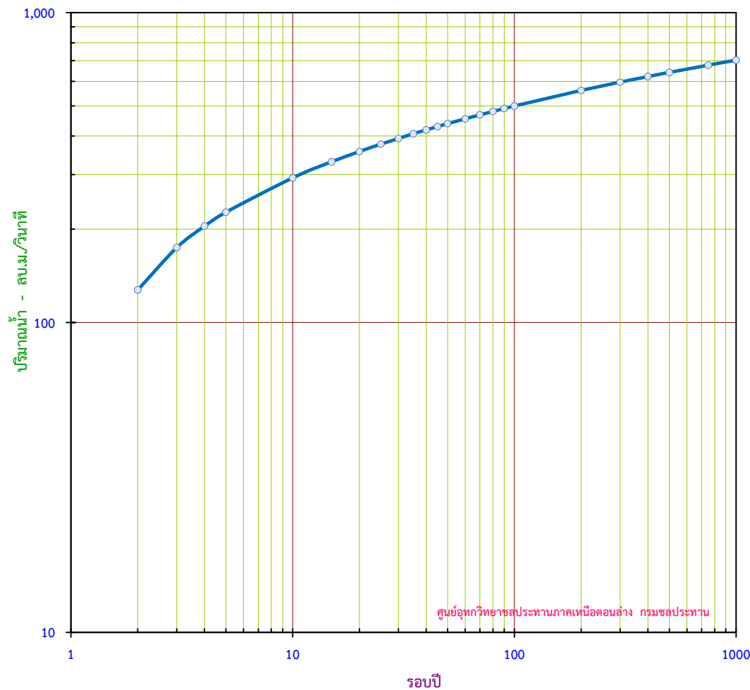
กราฟแสดง ปริมาณน้ำสูงสุดรายปี ขนาดรอบปีต่างๆ สถานี P.50A อ.โกสุมพินคร จ.กำแพงเพชร
